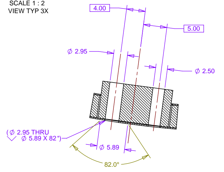
DETAIL D SCALE 4 : 1 VIEW TYP 3X
